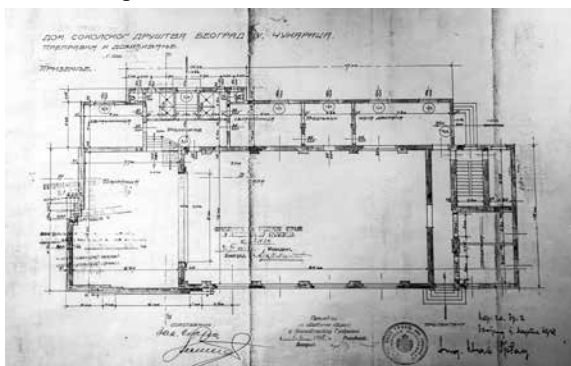
Слика 3 Иван Грбац, Соколски дом Београд IV, основа приземља, 1938. година (извор: ИАБ, ф–XX–13–1932)
