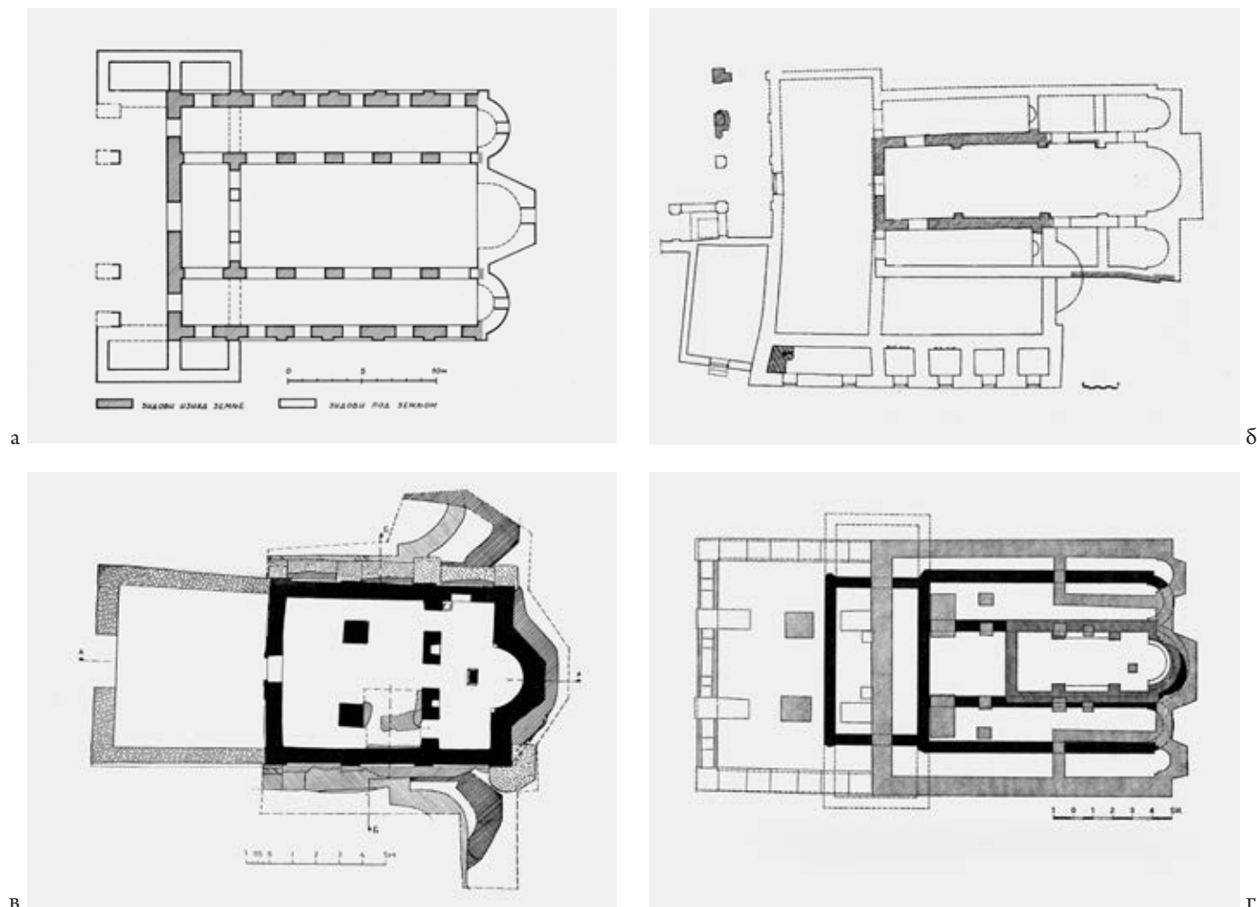
Сл. 179. Основе преднемањитких црква: а. Призрен, Богородица Љевишка; б. Пешка патријаршија, Свети апостоли; в. Липјан, црква Ваведења Богородичиног; г. Грачаница
