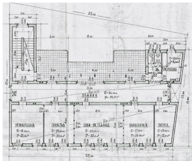
Сл. 7. Пројекат Обданишта Женској хришћанској њокреџи, арх. Милош Драгићиновић, 1938. (извор: Историјски архив Београда)
