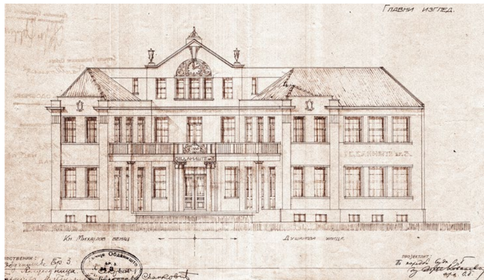
Сл. 5. Пројекат Обданишћа бр. 3, арх. Ђорђе Коваљевски, 1930–1931. (извор: Историјски архив Београда)
