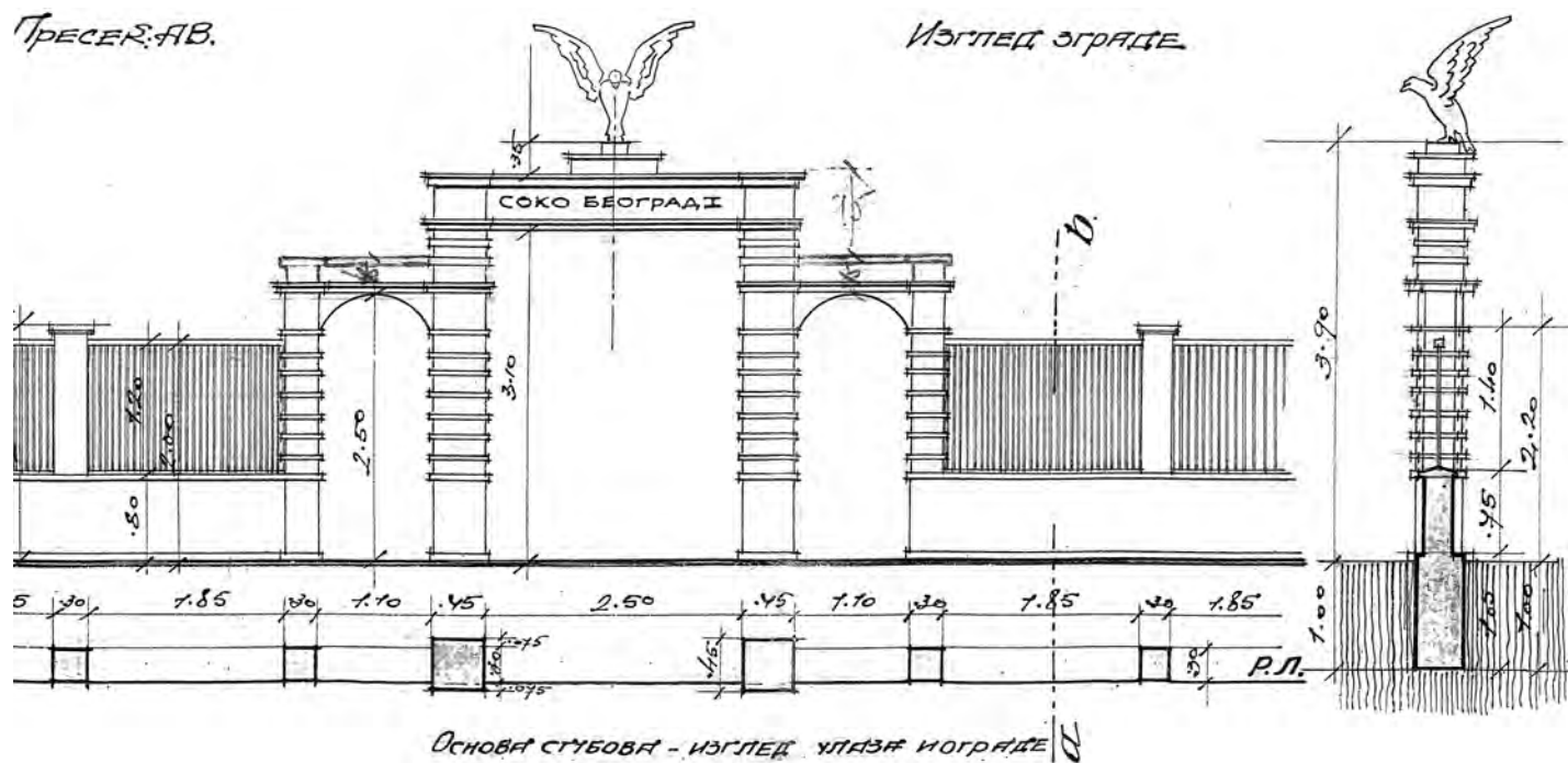
Сл. 4. Цвейко Анђелковић, Пројекат капије лейтнеј вежбалишћа Соколској групиња Београд I, 1932. (ИАБ, Ф37-53-1932)
