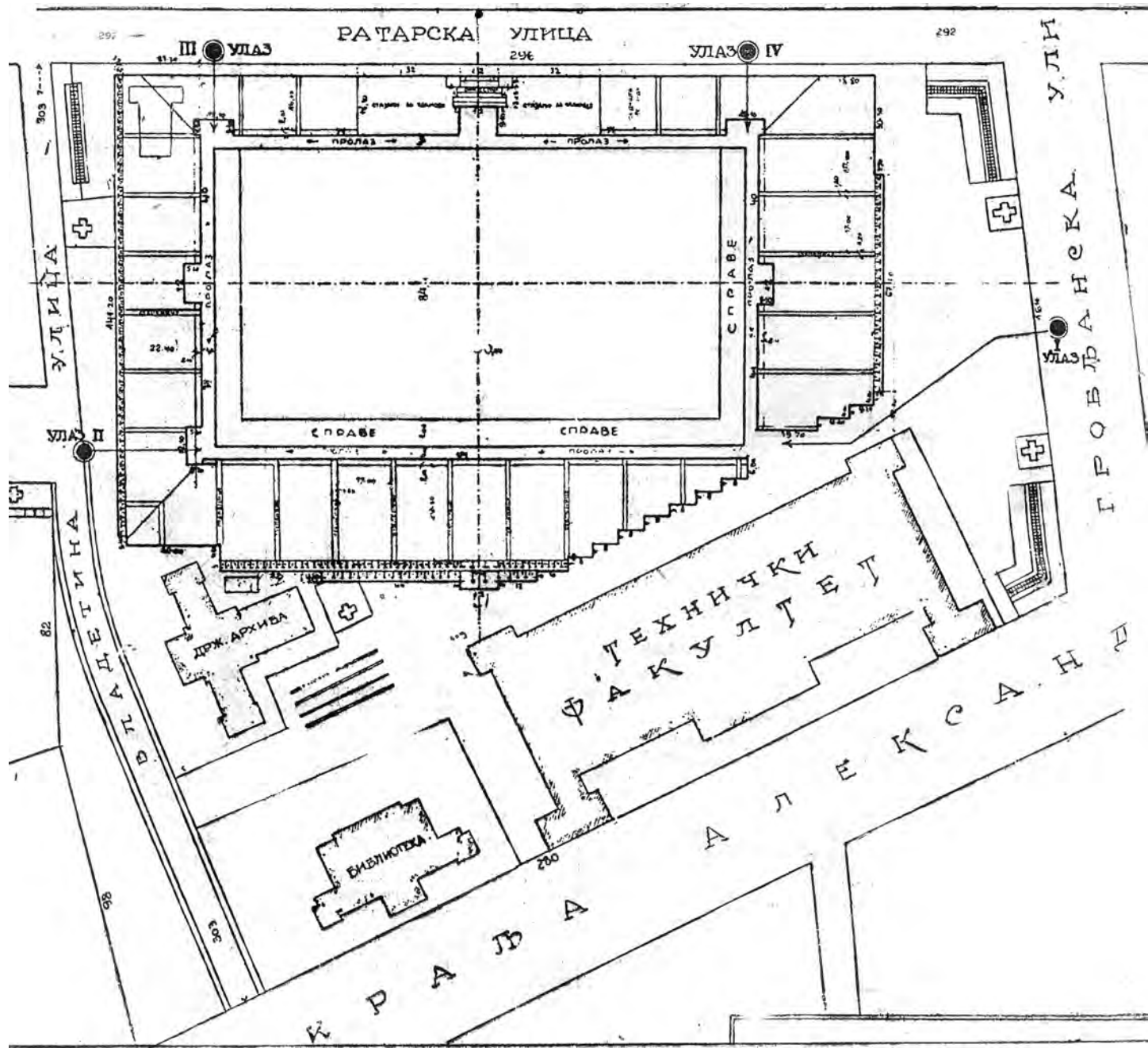
Сл. 8. Момир Коруновић, Пројекат Соколској стјадиона (Време, јануар 1930)
