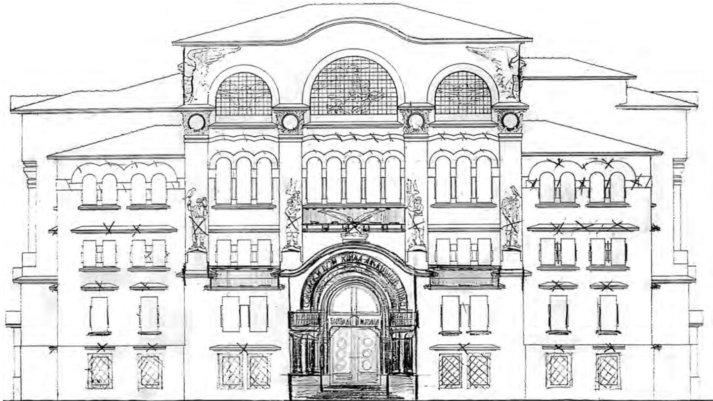
Сл. 1. Момир Коруновић, Пројекат Соколског дома „Матица“, 1933. (ИАБ, I-2a/1946)
