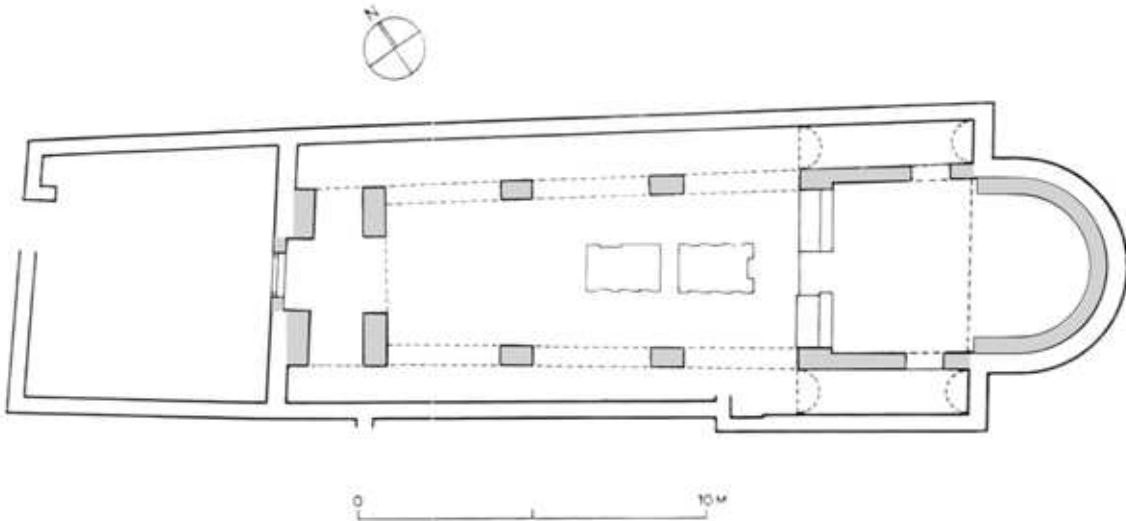
Сл. 1. Стон, Св. Марија на Горици (данас Св. Магдалена/„Мандаљена“), основа са обележеним накнадним средњовековним доградњама (према I. Fiskoviću, цртеж арх. Г. Толић).
