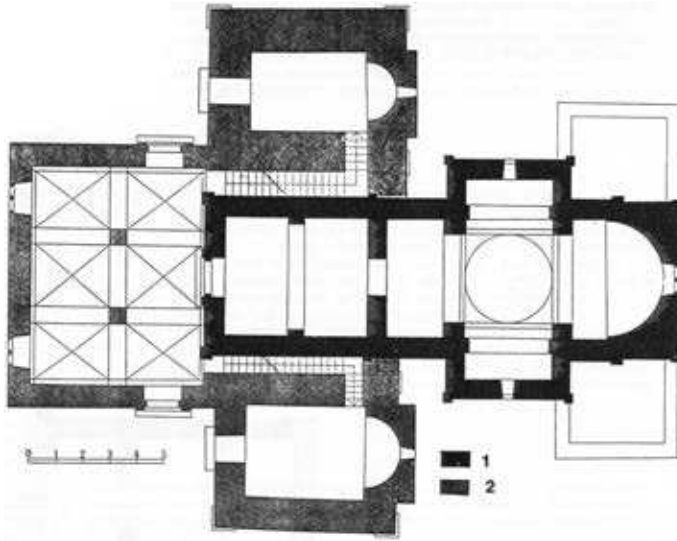
Сл. 6. Студеница Хвоштанска, основа (према В. Кораћу/ М. Чанак-Медић)
