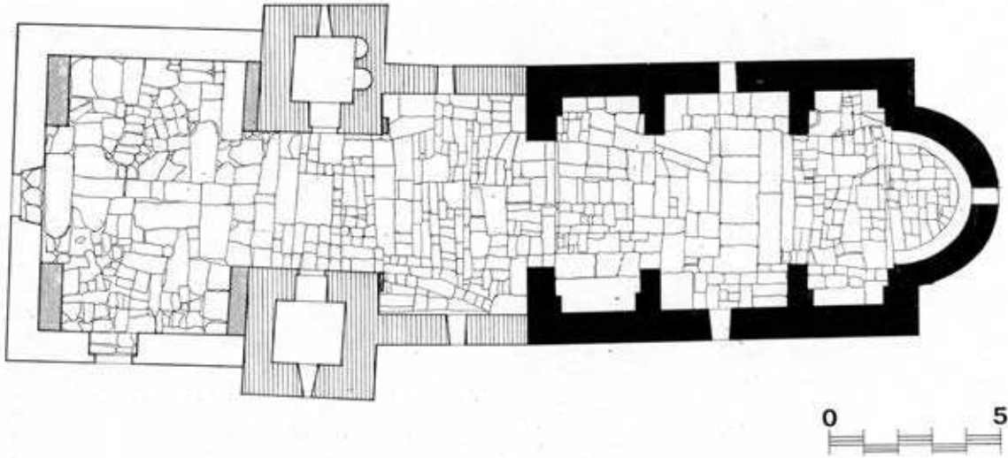
Сл. 2. Беране, Св. Ђорђе, основа (према М. Чанак-Медић).
